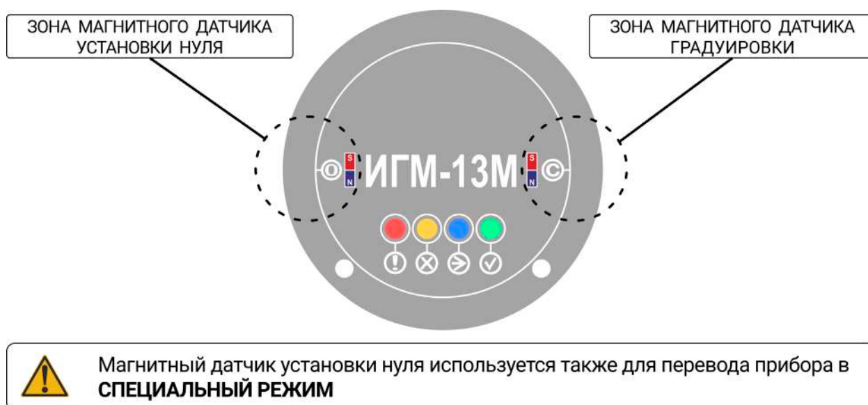
Рисунок К.1 - Расположение магнитных датчиков
