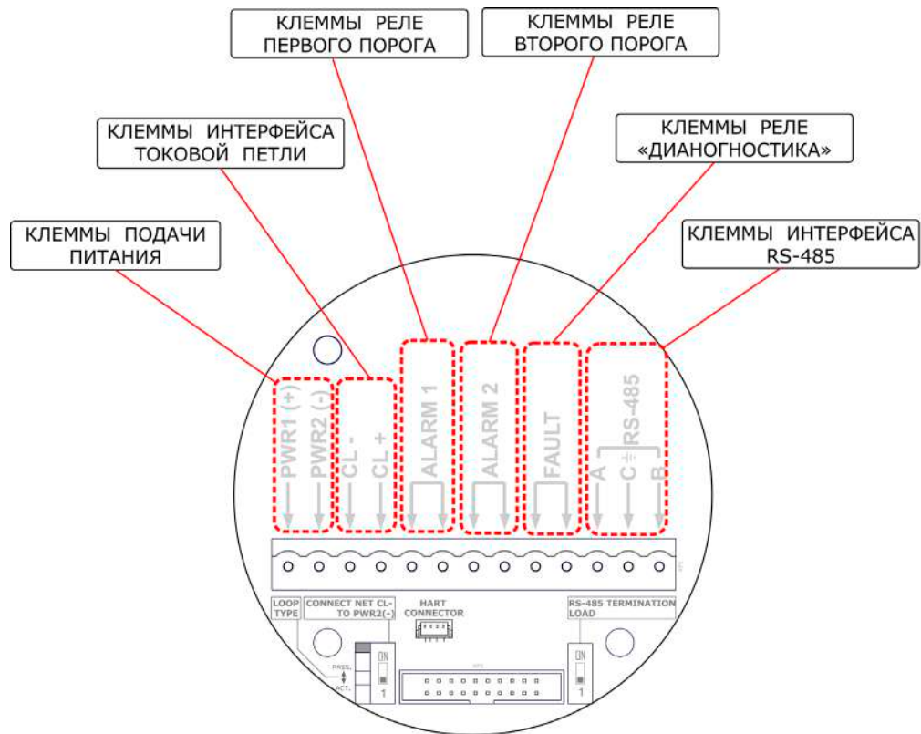
Рисунок 12 – Функциональное назначение клемм подключения внешних электрических цепей ИГМ-13М, изготовленных с апреля 2023г.
