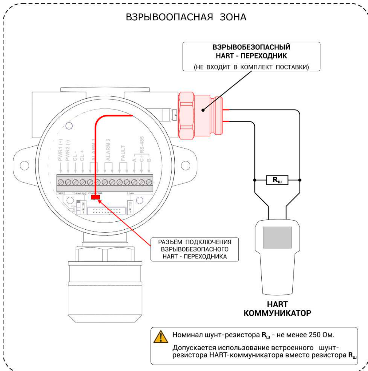
Рисунок И.6 – Подключение взрывобезопасного HART-переходника для подключения коммуникаторов во взрывоопасной зоне
