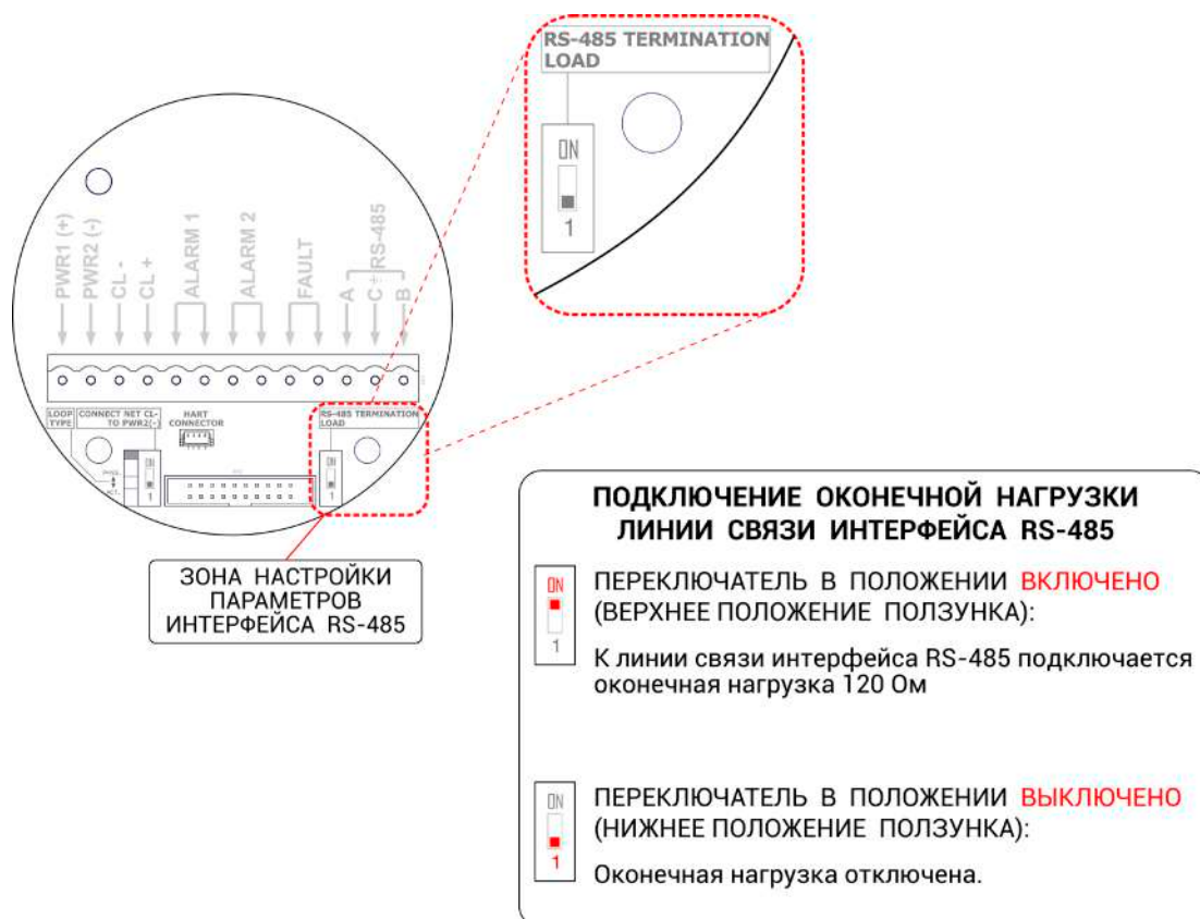
Рисунок 28 – Подключение оконечной нагрузки линии связи интерфейса RS-485 для ИГМ-13М, изготовленных с апреля 2023г.
