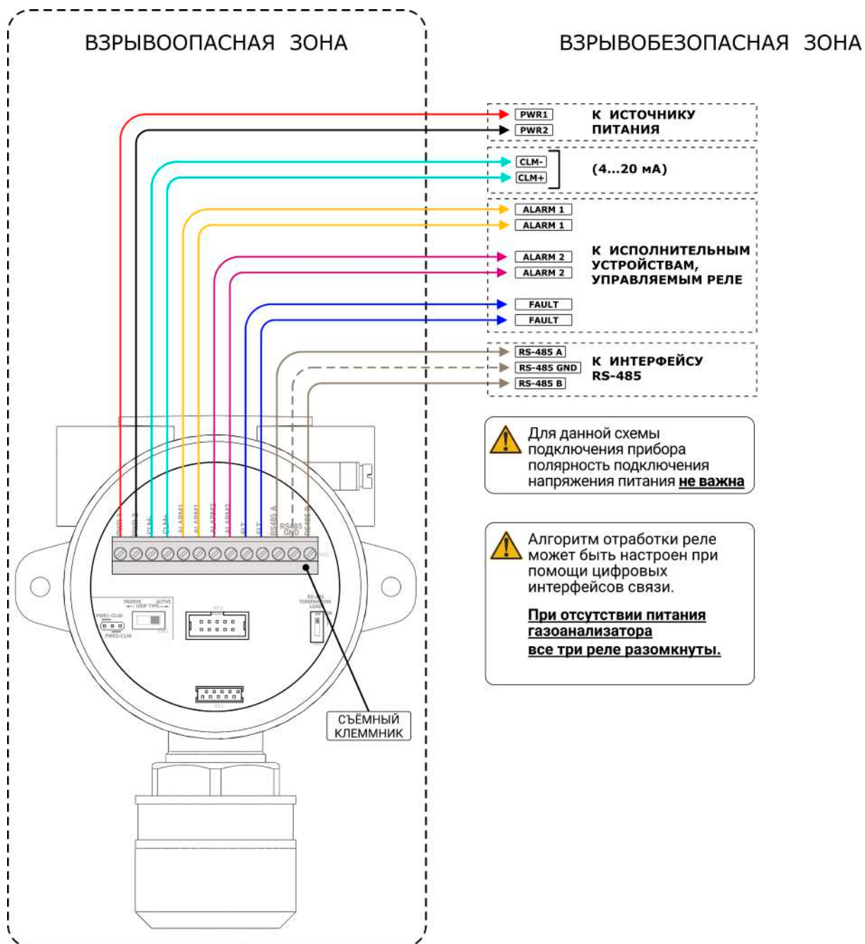
Рисунок 3.15 – Одновременное подключение к ИГМ-13М по интерфейсам токовой петли, RS-485 и реле
