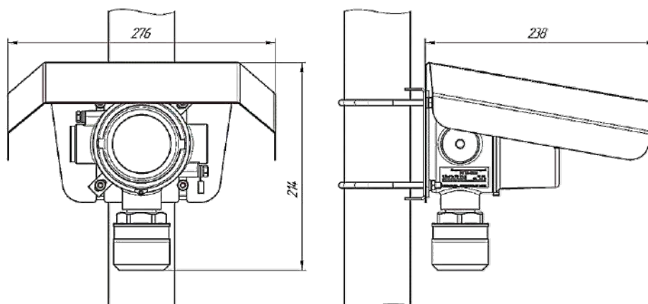
Рисунок 21 – Габаритные размеры ИГМ-13М (корпус тип 3) совместно с установленным защитным козырьком
