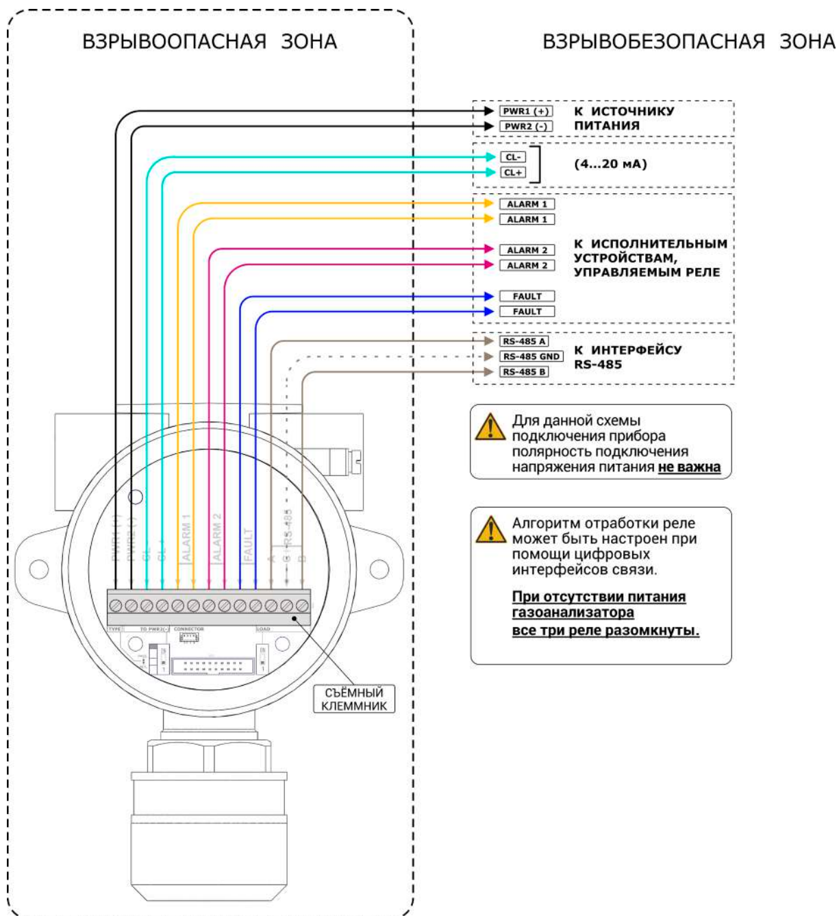
Рисунок И.9 – Одновременное подключение к ИГМ-13М по интерфейсам токовой петли, RS-485 и реле
