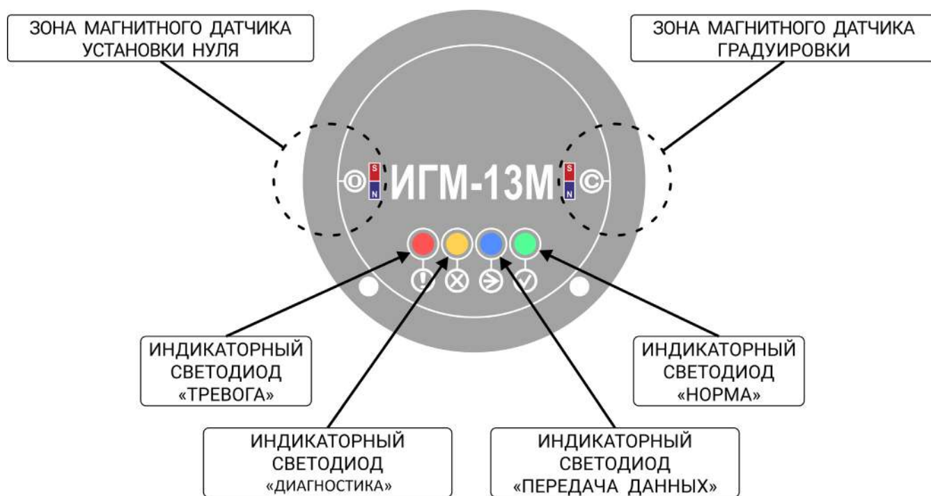
Рисунок 9– Лицевая панель ИГМ-13М
