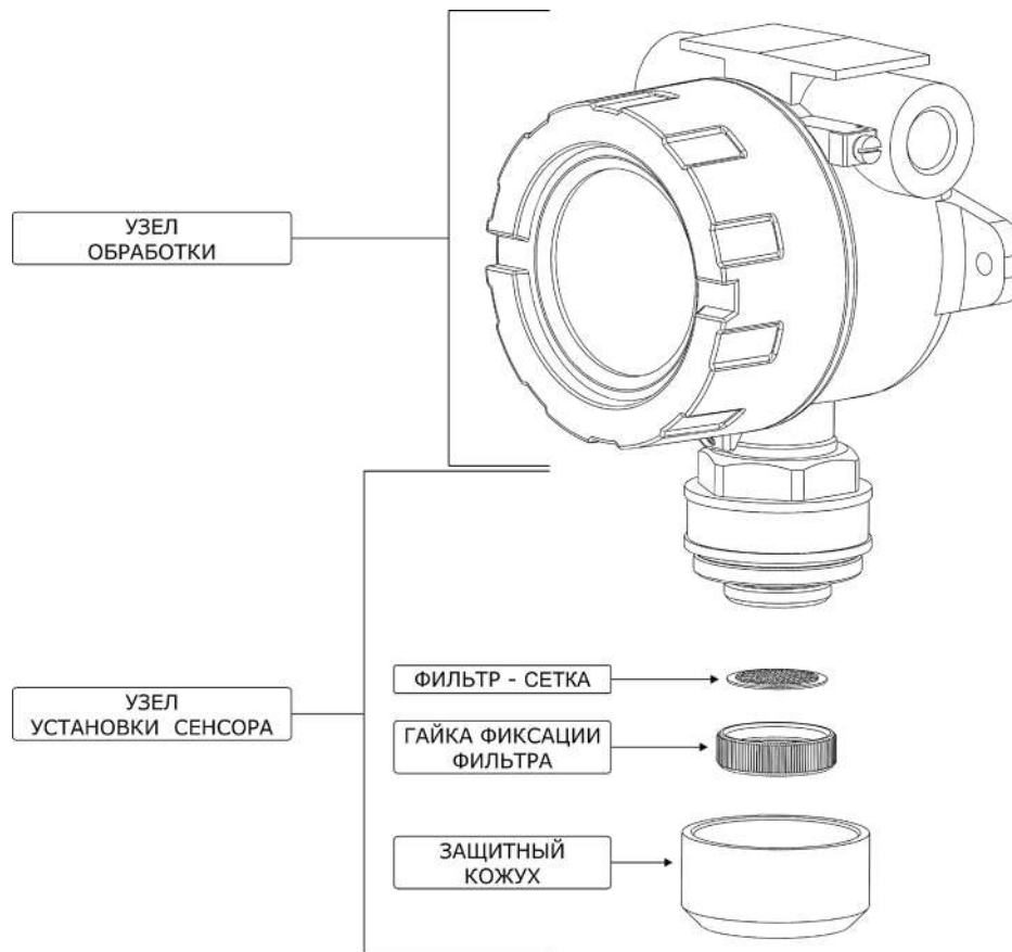
Рисунок 7 – Основной функциональный состав ИГМ-13М
