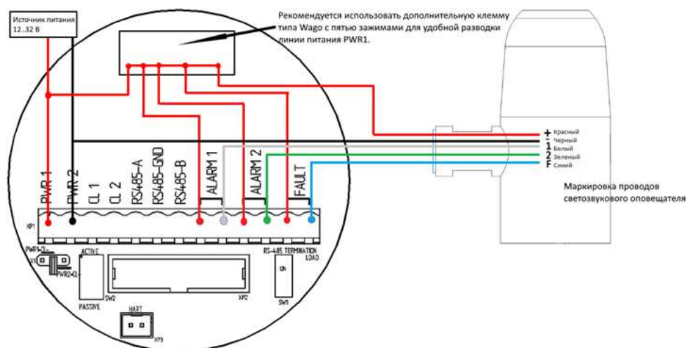
Рисунок 22 – Схема подключения светозвукового сигнализатора ЭМИ-СЗ к ИГМ-13М, изготовленным до апреля 2023г.
