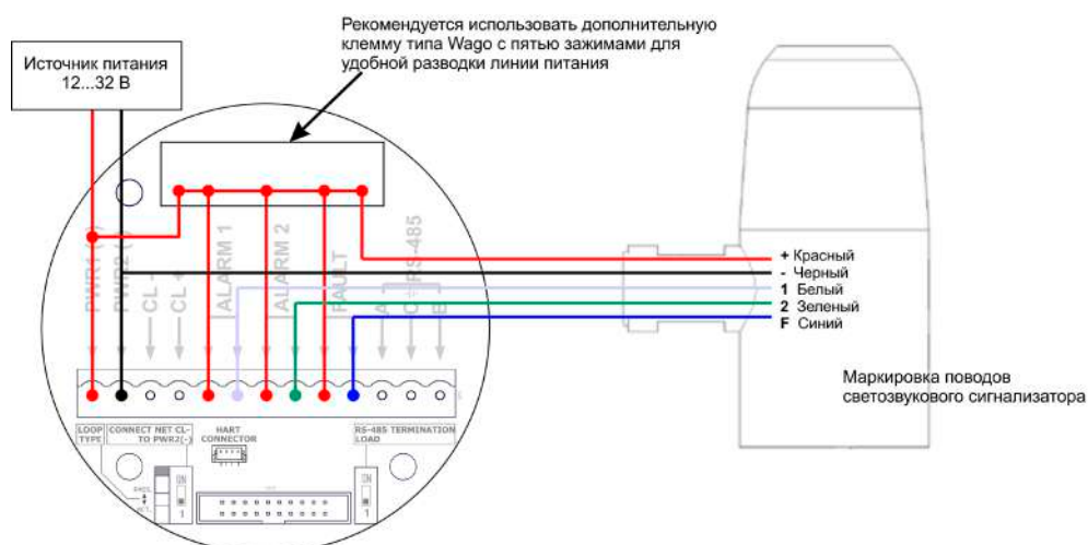
Рисунок 23 – Схема подключения светозвукового сигнализатора ЭМИ-СЗ к ИГМ-13М, изготовленным с апреля 2023г.
