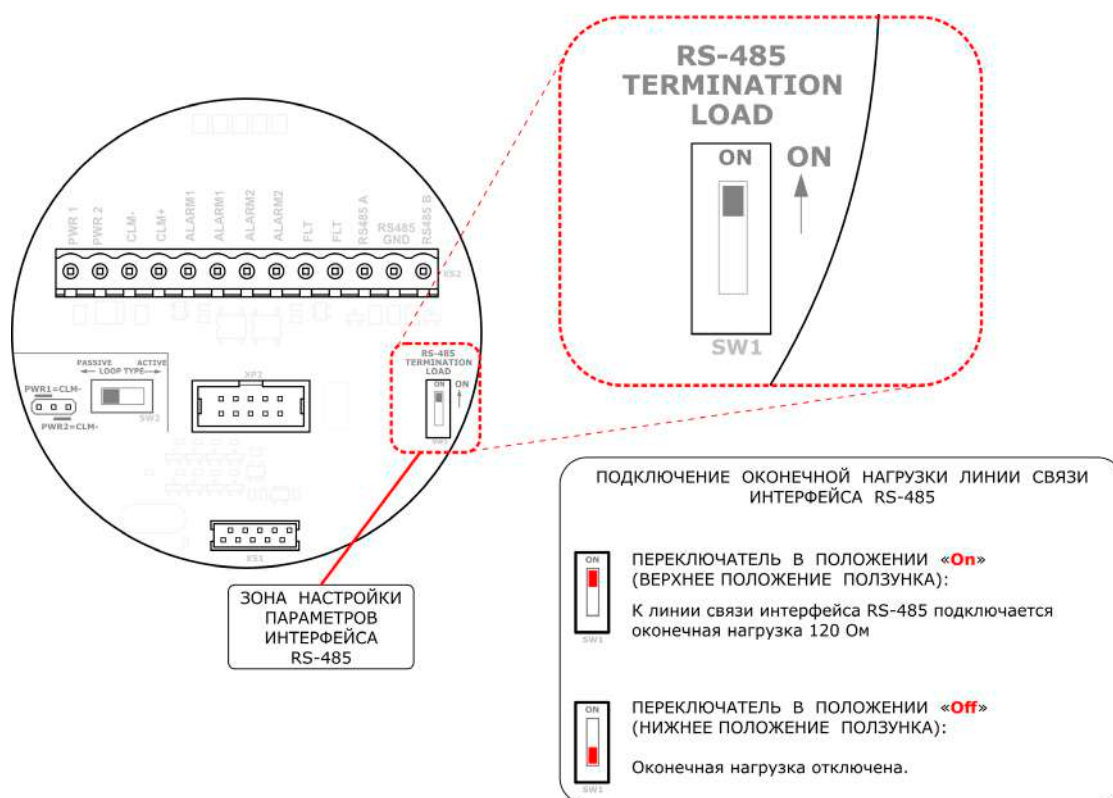
Рисунок 27 – Подключение оконечной нагрузки линии связи интерфейса RS-485 для ИГМ-13М, изготовленных до апреля 2023г.
