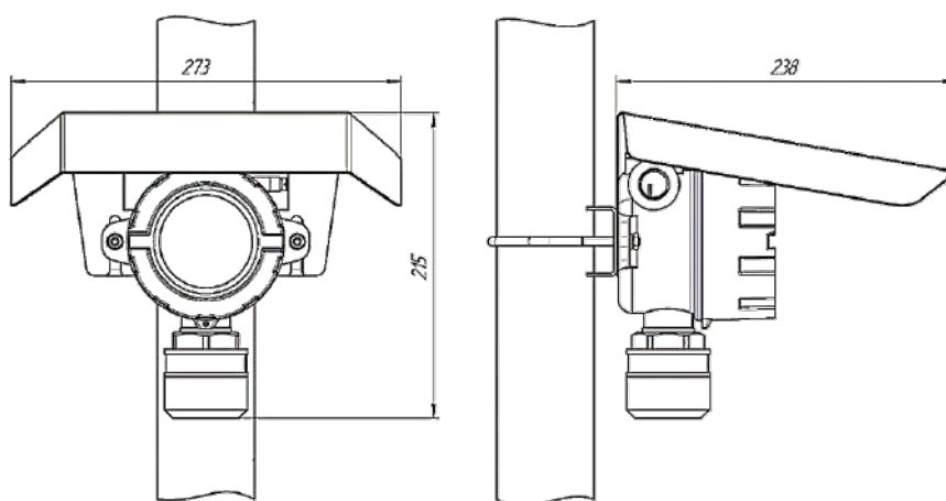
Рисунок 20 – Габаритные размеры ИГМ-13М (корпус тип 1) совместно с установленным защитным козырьком
