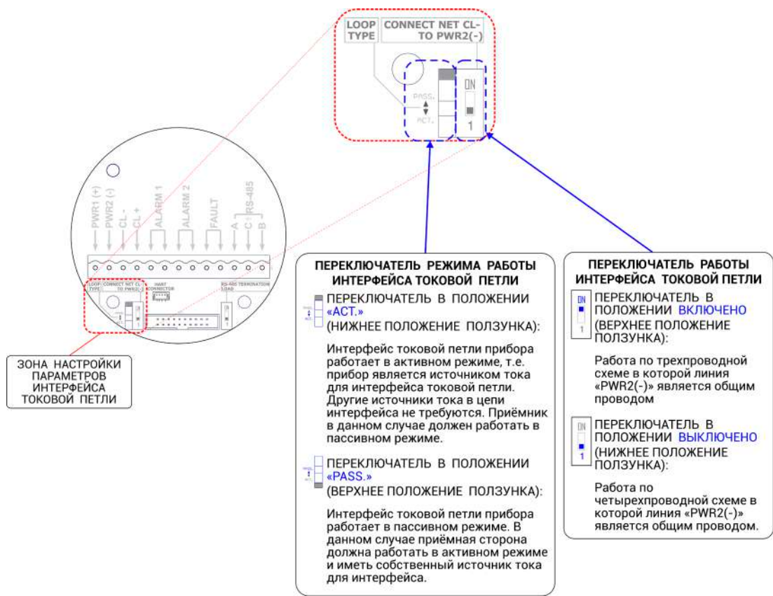
Рисунок 26 – Настройка параметров интерфейса токовой петли для ИГМ-13М, изготовленных с апреля 2023г.
