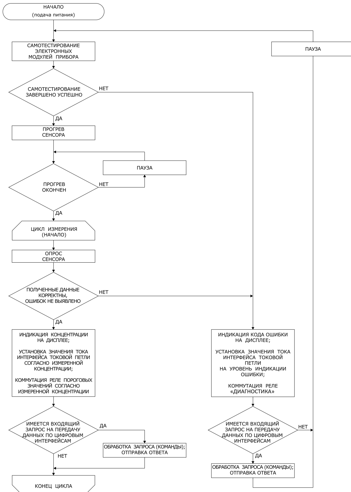
Рисунок 14 – Алгоритм функционирования ИГМ-13М
