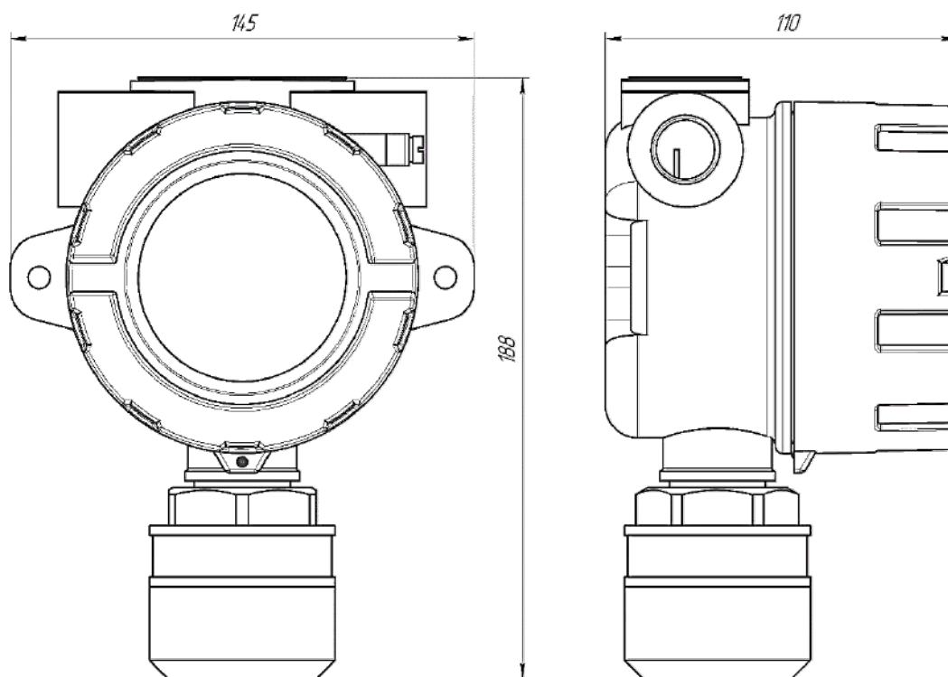
Рисунок 5 – Габаритные размеры ИГМ-13М (корпус тип 1)
