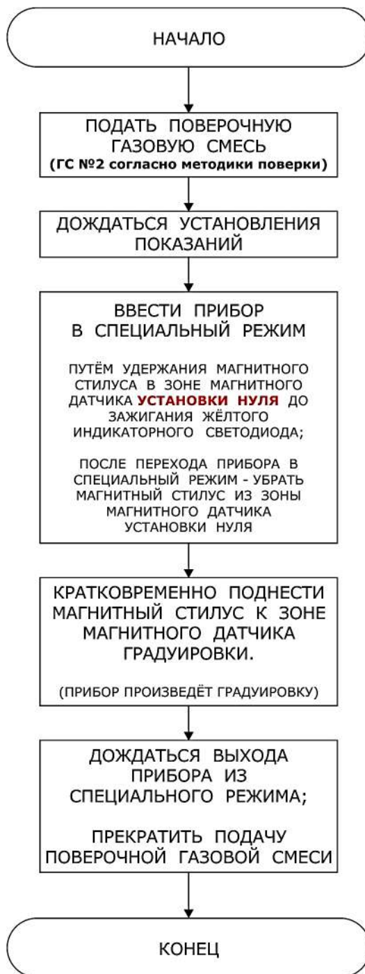
Рисунок К.2.1 - Алгоритм градуировки чувствительности по концентрации при помощи магнитного интерфейса
